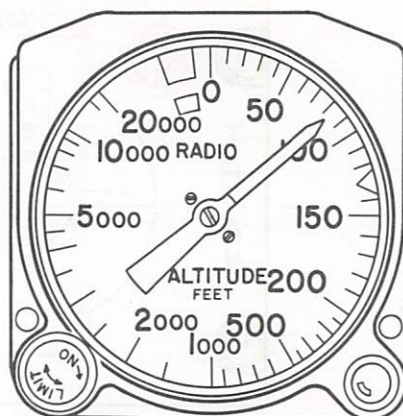
APN-22 INDICATOR
