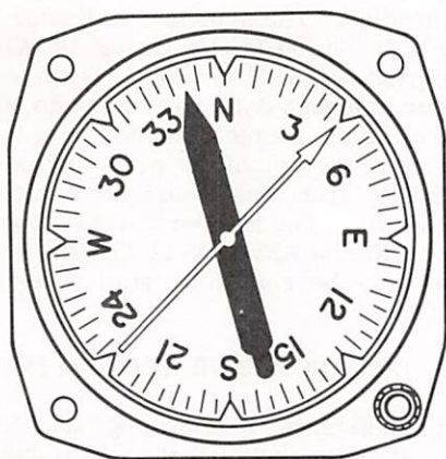
RMI
