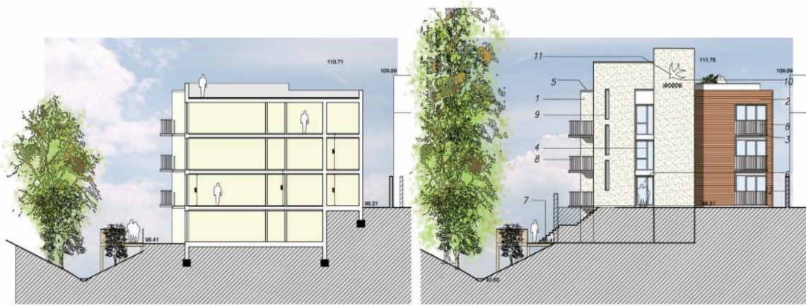
SECTION A-A SCALE 1:200 @ A3
