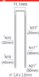
Agrafes série 700 Agrafes série S15
