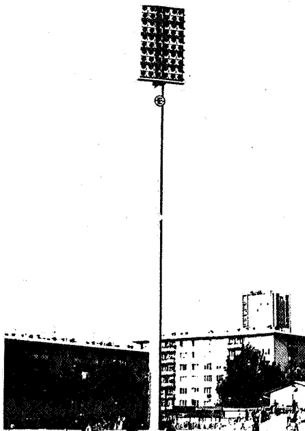
Jedan od četiri reflektora na stadionu Grbavica
