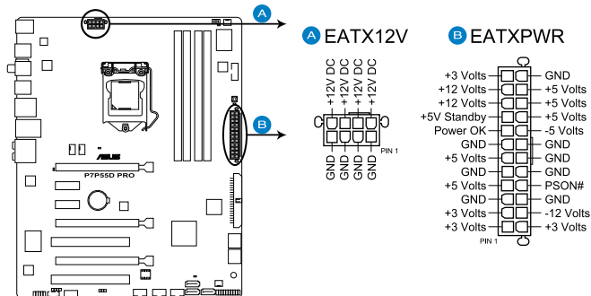
Connecteurs d'alimentation de la P7P55D PRO
