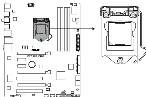
Socket 1156 de la P7P55D PRO
