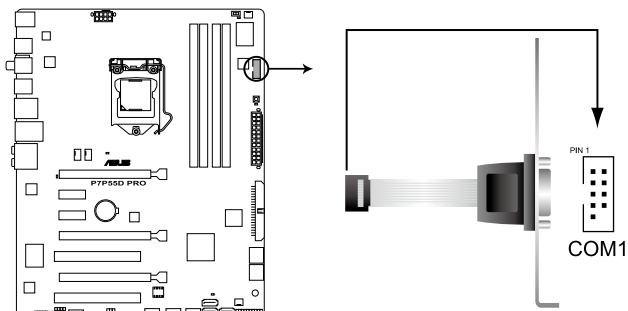
Connecteur COM de la P7P55D PRO
