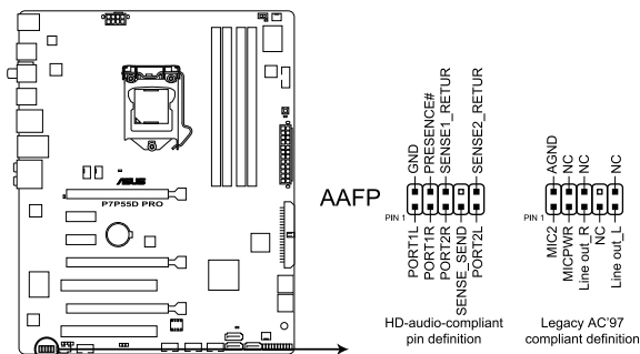
Connecteur pour port audio en façade de la P7P55D PRO
