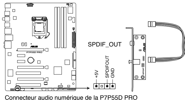
Connecteur audio numérique de la P7P55D PRO
