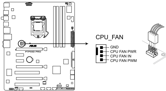
Connecteur CPU_FAN de la P7P55D PRO
