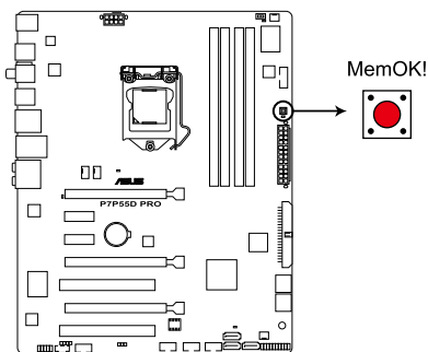
Interrupteur MemOK! de la P7P55D PRO
