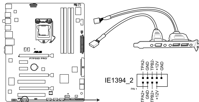
Connecteur port IEEE 1394a de la P7P55D PRO
