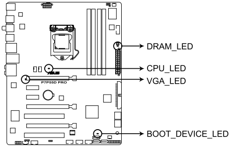
Voyants d'état du POST de la P7P55D PRO
