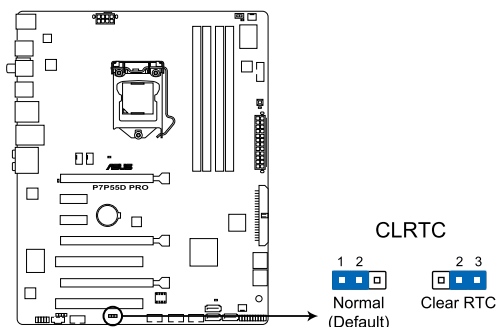
Jumpers d'effacement de la mémoire RTC de la P7P55D PRO
