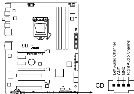
Connecteur audio pour lecteur optique de la P7P55D PRO
