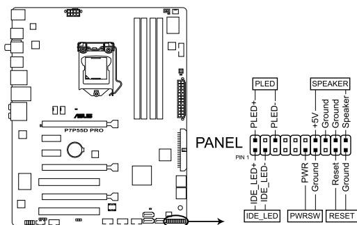
Connecteurs panneau système de la P7P55D PRO
