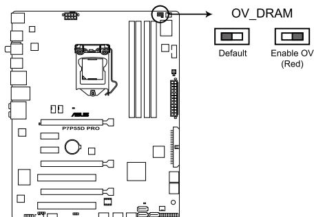
Interrupteur de surtension de la P7P55D PRO
