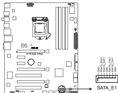
Connecteurs SATA E1 de la P7P55D PRO
