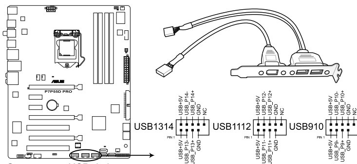
Connecteurs USB de la P7P55D PRO
