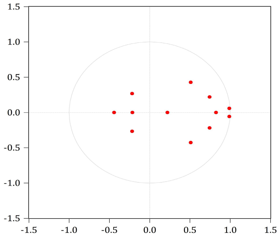
Διάγραμμα Π-1: Ιδιοτιμές του SVAR υποδείγματος
