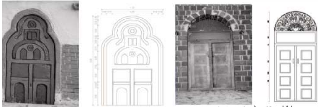
(191) باب مستخدم في مبنى حديث (عرض الضلعة 90سم وطول 185سم (192) باب مسجد قباء (عرض 117 سم وطول 200سم) [التراث المعماري للمدينة نقلاً عن التاريخ والعمارة] [التراث المعماري . ص 8 نقلاً عن متحف دار المدينة للتراث]
